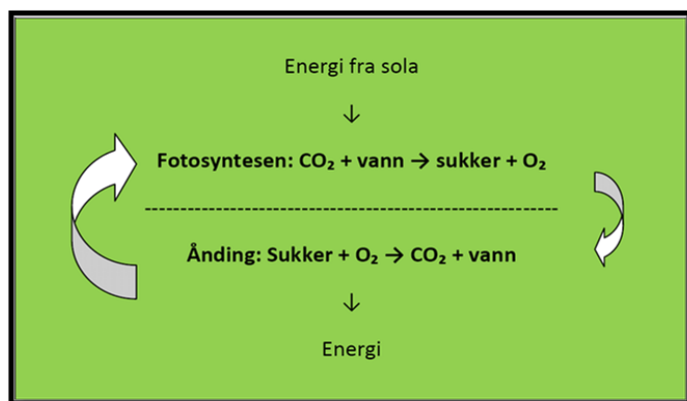
Figur: Ubalansen i karbonets kretsløp - sterkt forenklet og skjematisk
